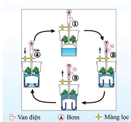
Hình 1: cấu tạo và nguyên lý hoạt động của bình RITA
