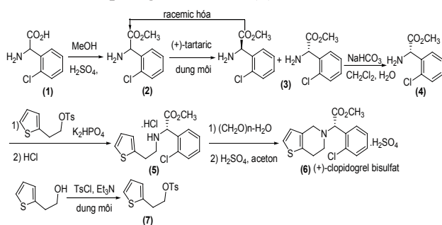
Sơ đồ tổng hợp (S)-clopidogrel bisulfat
